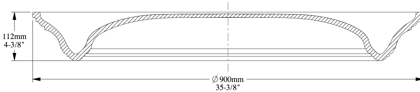
SECTION A-A
