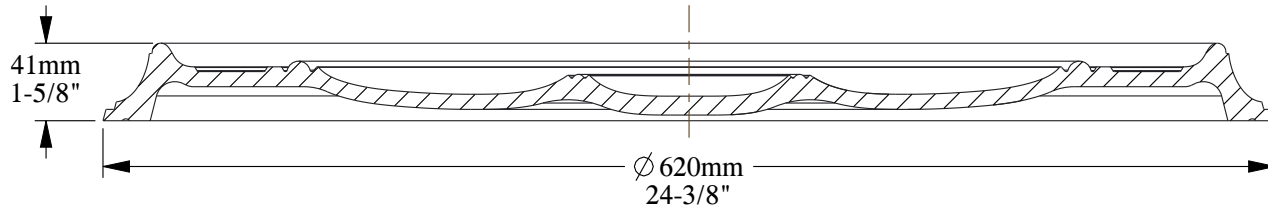
SECTION A-A
